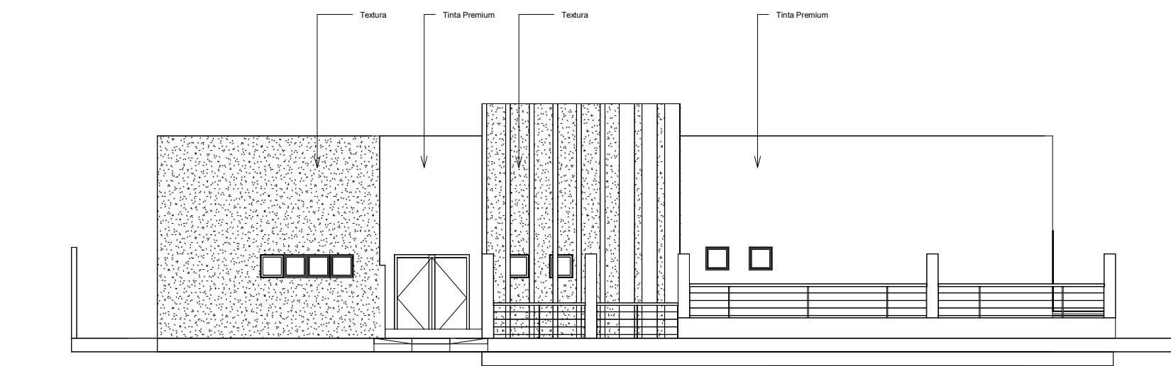
2 FACHADA 1 : 100
